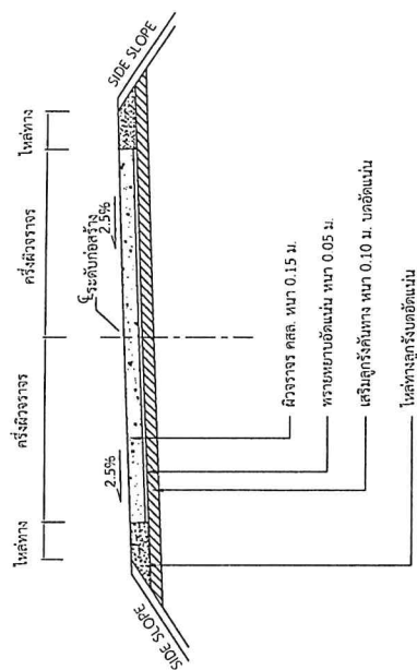
รูปตัดแสดงโครงสร้างถนนคอนกรีตเสริมเหล็กและคุณสมบัติวัสดุ
